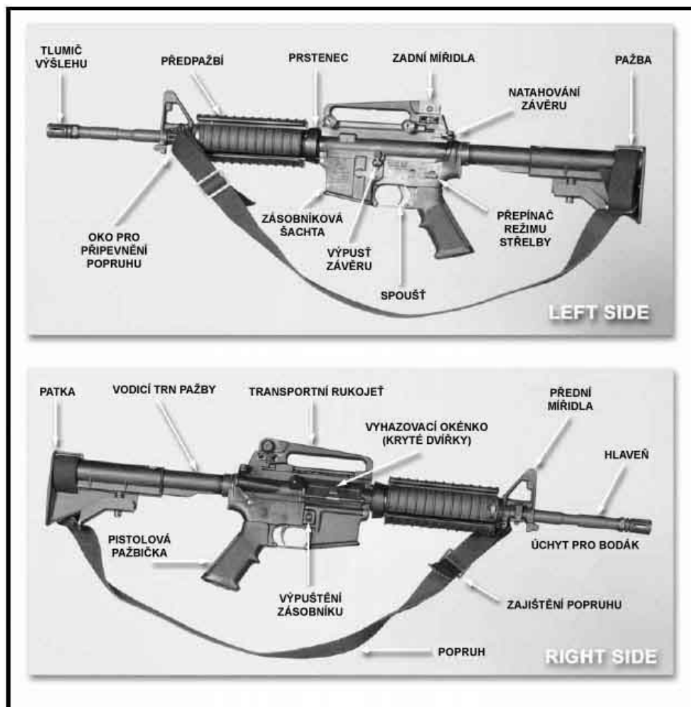
Obr. A. Nomenclature, M4-series carbine (M4 - popis)
